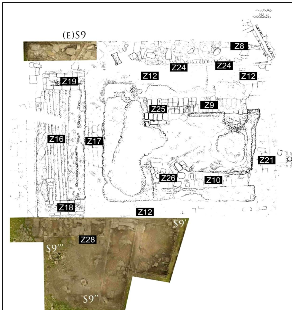
Fig. 2. Substrucția podium-ului și elementele stylobatului (după Piso, CCA. Campania 2016, 2017, p. 7).
